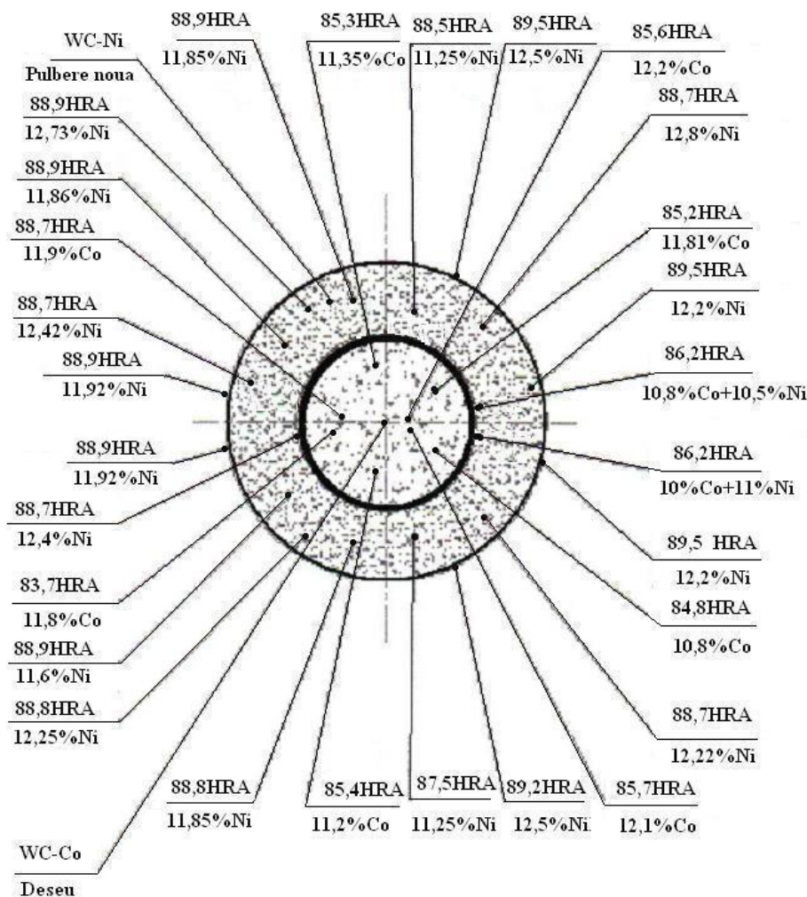
Figure 2. Ball made in multi-layer system. Slika 2. Kuglica napravljena iz višeslojnog sistema
